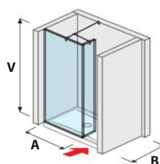
sklenená stena PURE vrátane krátkeho skla 70, 80 cm
