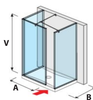
sklenená stena/walk in PURE do priestoru pre sprchovú vaničku 70, 80 × 80 cm | 70, 80 × 90 cm
