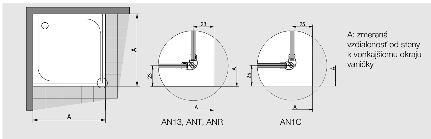
Obr. 1: Pri montáži na vaničku je pre AN13, ANT, ANR odsadenie 23 mm, pre AN1C 25 mm.
