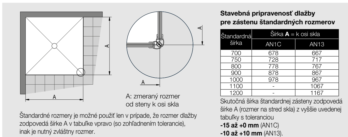
Obr. 2: Pri montáži na dlažbu sa pri výrobe nezohľadňuje žiadne odsadenie.
