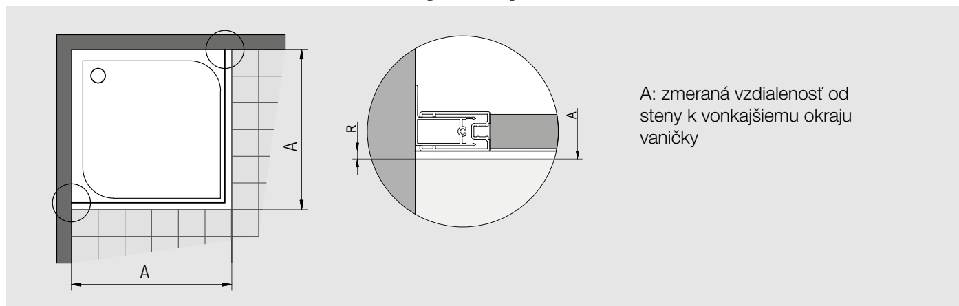
Obr. 1: U montáže na vaničku je odsadenie R závislé na veľkosti rádia vonkajšej hrany vaničky a je rovnaké pre štandardné i zvláštne rozmery (pozri detail 1).
