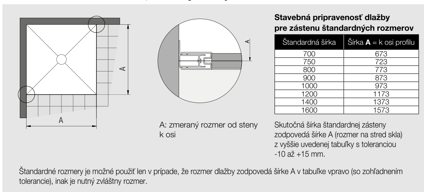
Obr. 2: Pri montáži na dlažbu sa pri výrobe nezohľadňuje žiadne odsadenie.
